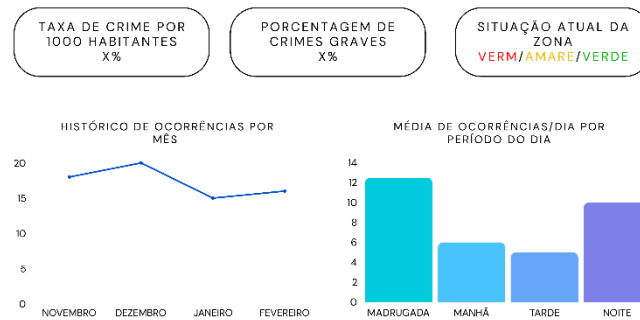
Figura 9 - WF03
