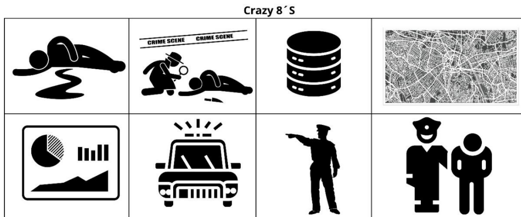
Figura 3 - Crazy 8
